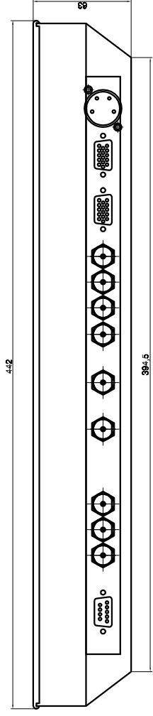
Ansicht von unten (ohne Bügel)
